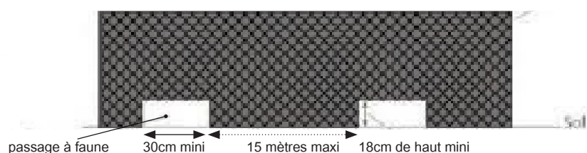
PASSAGE À FAUNE POUR LES MURS ET MURETS
